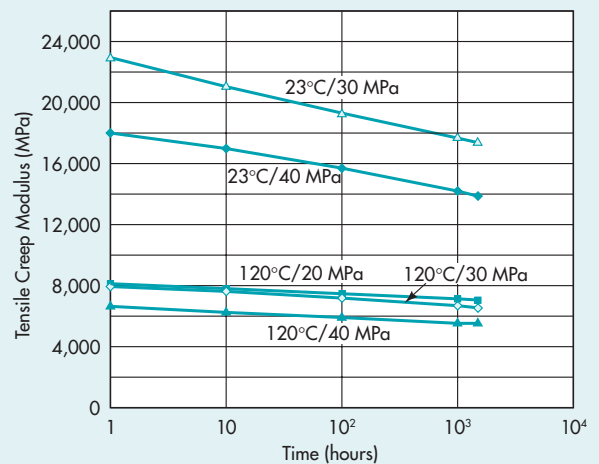
Fig. 3.1.12 • Tensile Creep Modulus, Vectra H140
