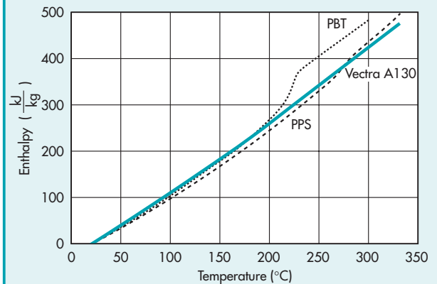
Fig. 3.2.13 • Enthalpy
